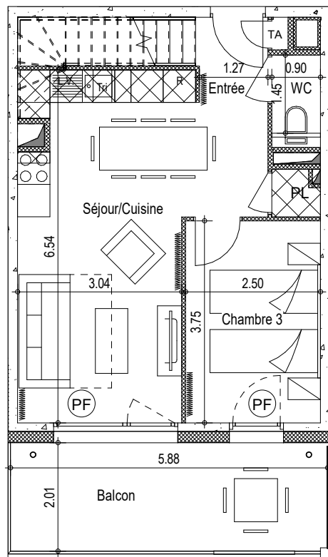
Duplex niveau b R+5
